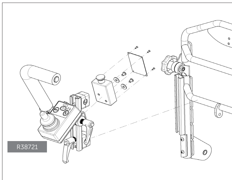
1. Samlingsveilede - Nødstopp på ledsagerstyring
