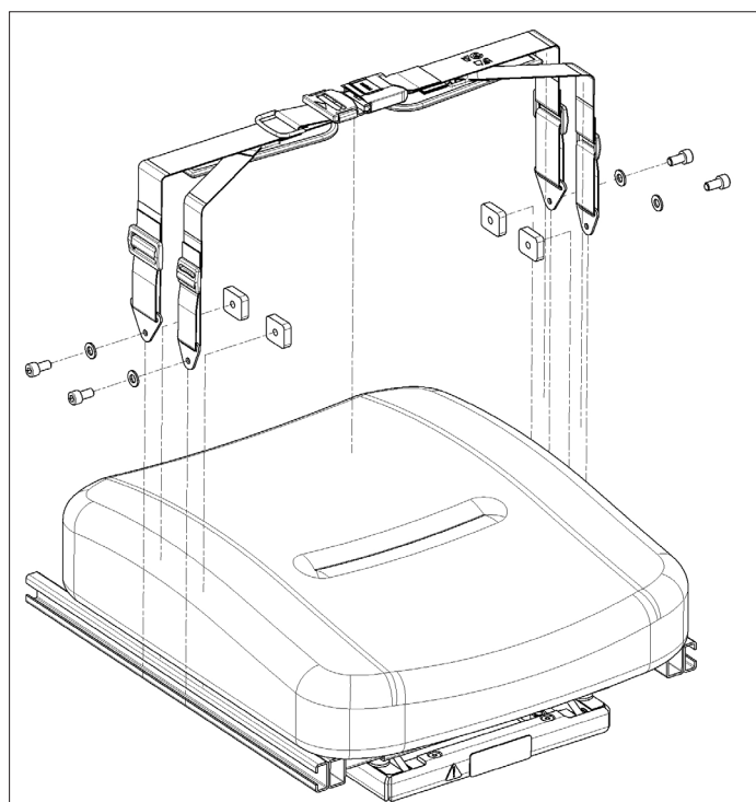
1. Samlingsveilede - Y-sele
