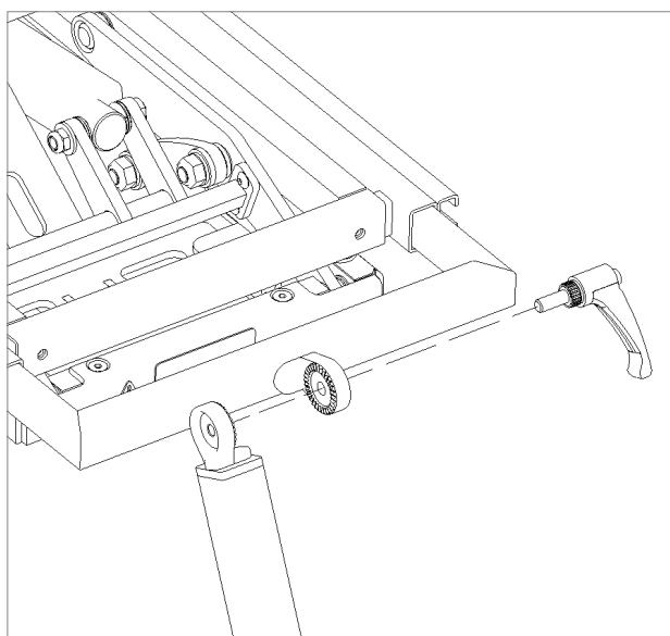
1. Samlingsveilede - fotplateoppheng
