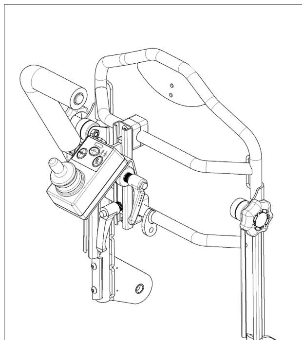
2. Ledsagerstyring montert
