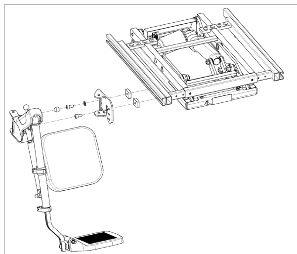
1. Samlingsveilede - Benstøtte gas, med utsving
