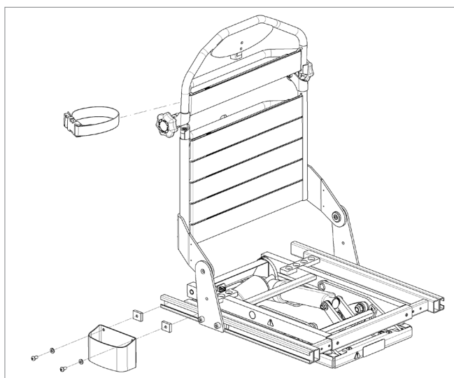
1. Samlingsveilede
