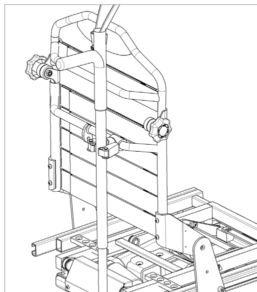
2. Krykkeholder montert på rygg
