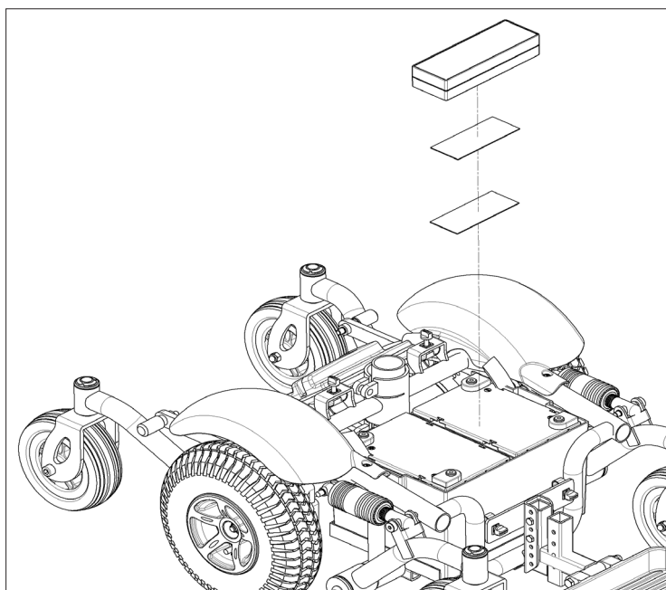
1. Samlingsveilede - Bryterpanel for rygg
