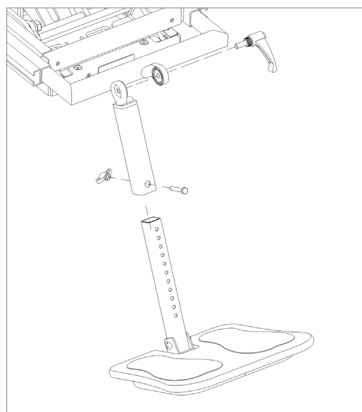
2. Montering av fotplate
