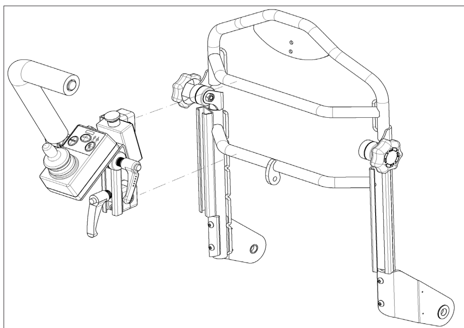
1. Samlingsveilede - Ledsagerstyring komplett
