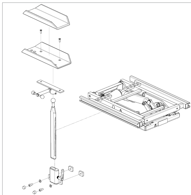
1. Samlingsveilede
