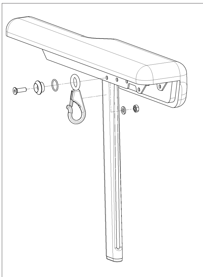
1. Samlingsveilede - Karabinkrok
