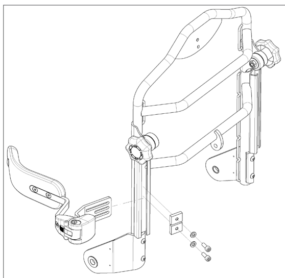
1. Samlingsveilede - Sidestøtte lår
