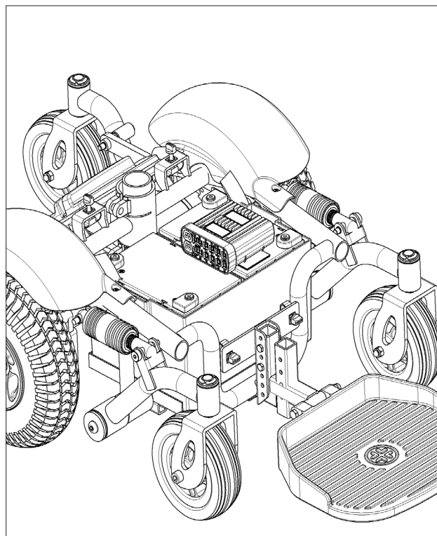
2. Aktuatormodul montert
