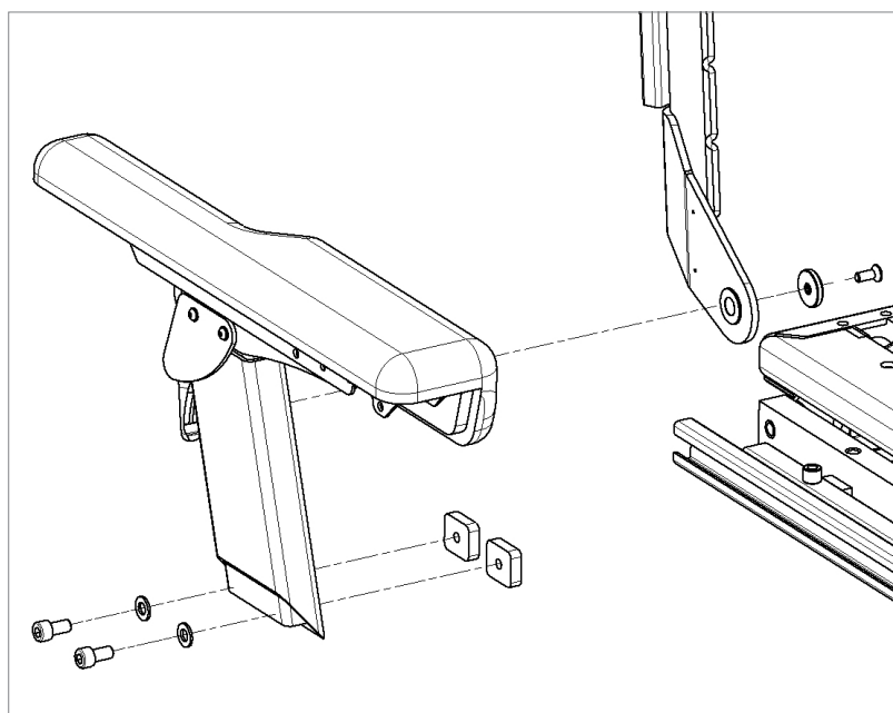
1. Samlingsveilede - Vinkelpute
