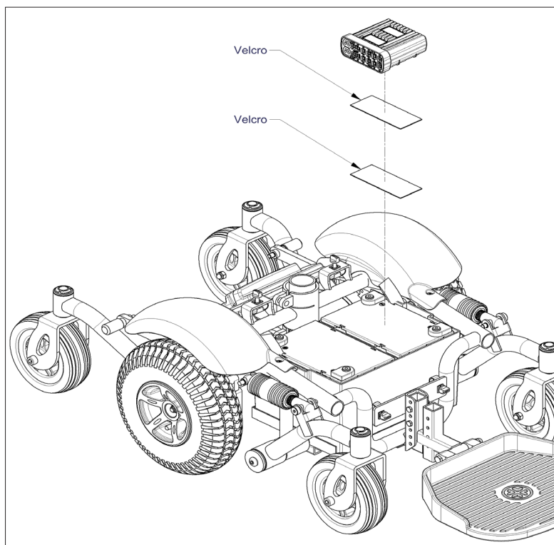
1. Samlingsveilede - Aktuatormodul på karosseri
