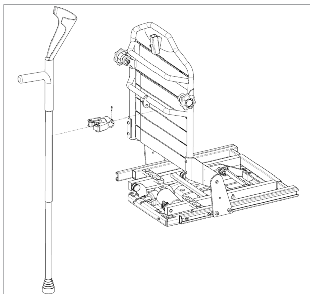
1. Samlingsveilede - Krykkeholder
