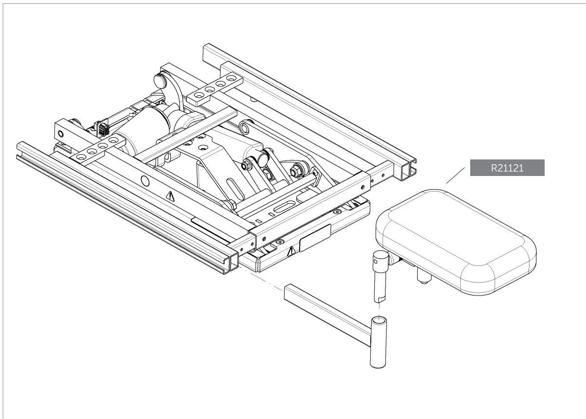
2. Samlingsveilede - Amputationsstøtte
