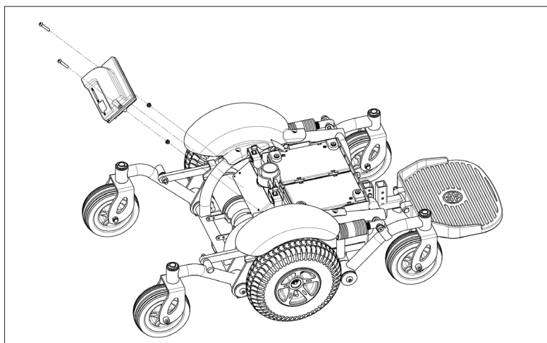
1. Samlingsveilede - powermodul
