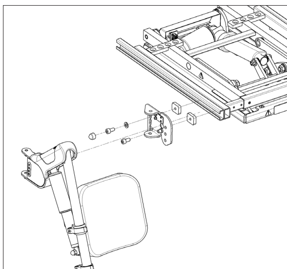
1. Samlingsveilede - Benstøtte el, med utsving
