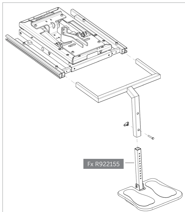
1. Samlingsveilede - oppheng og fotplate
