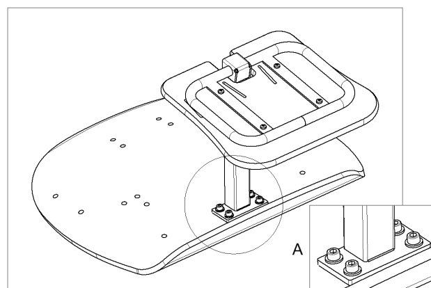
3. Fotplate påsat sæde
