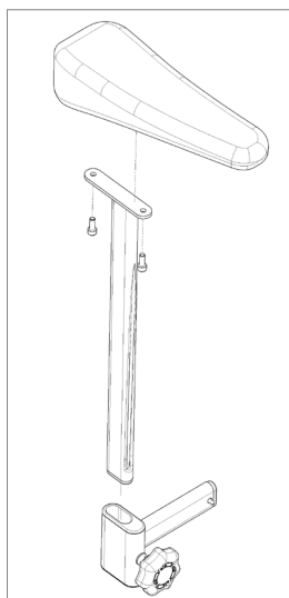
1. Samlingsveilede
