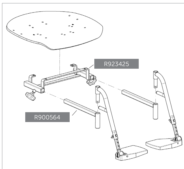
1. Samlingsveilede - Benstøtte udsving
