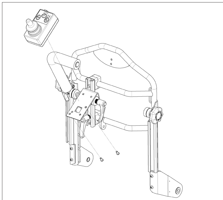
1. Samlingsveilede - Ledsagerstyring
