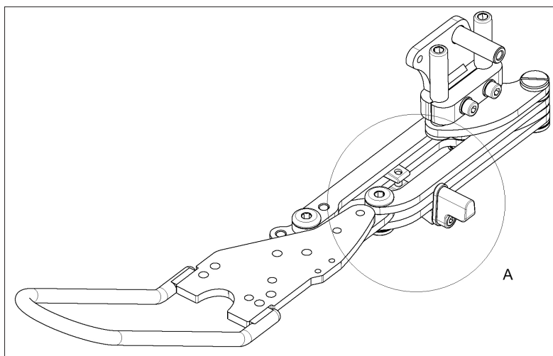
1. Samlingsveilede - Lås
