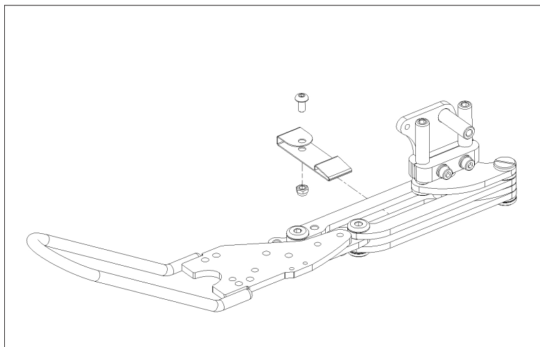
1. Samlingsveilede - Lås
