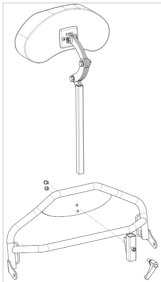
1. Samlingsveilede - Nakkestøtte
