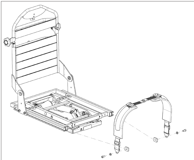
1. Samlingsveilede - Belte
