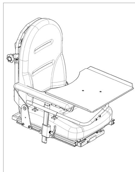
2. Samlet
