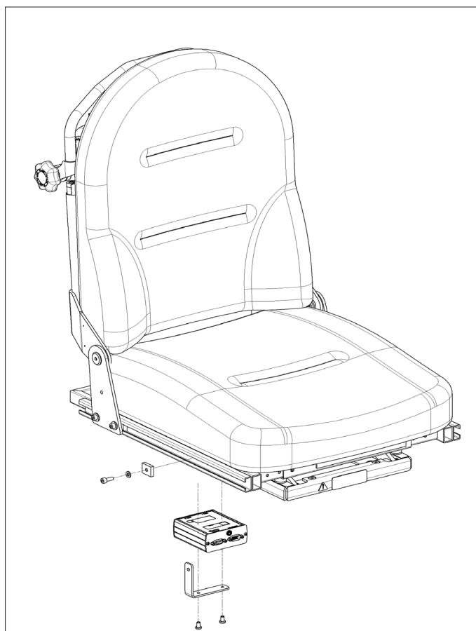
1. Samlingsveilede - Input/Output Modul på sete
