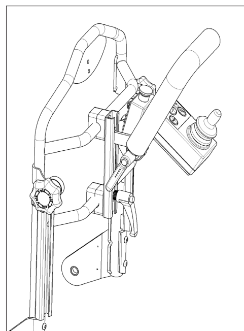
2. Ledsagerstyring montert
