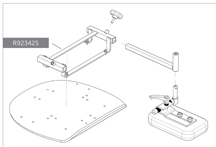
1. Samlingsveilede - Amputationsstøtte
