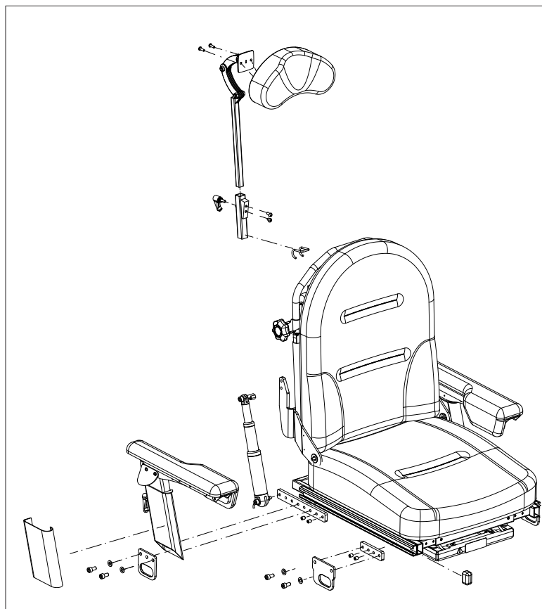
1. Samlingsveilede
