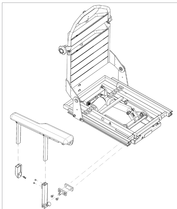
1. Samlingsveilede
